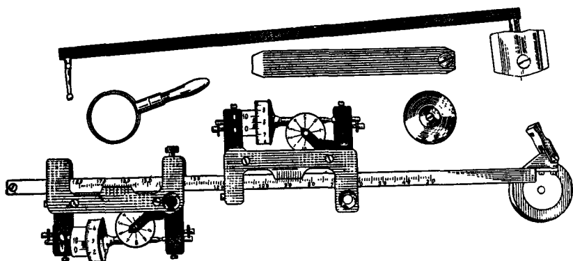
Рис. 27. Планиметр.
